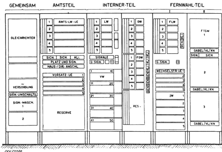
Gestellaufbau der genormten EW-Telephonanlage
