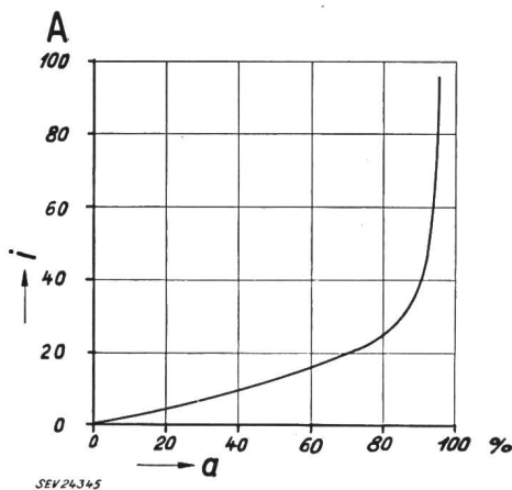
Fig. 3 Courbe d'étalonnage de l'amplificateur à valeur instantanée en A du courant mesuré
