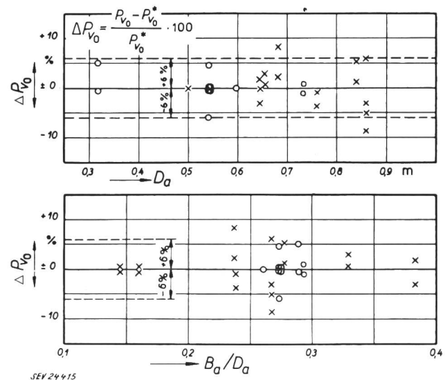
Fig. 40 Vergleich der Rechnungsergebnisse P_{v_0} nach den Formeln (17) und (18) und nach Hilfsdiagramm Fig. 39 mit den Versuchsergebnissen P_{v_0}^* (unverschaltete Räder) ○ einteilige Räder × mehrteilige Räder
