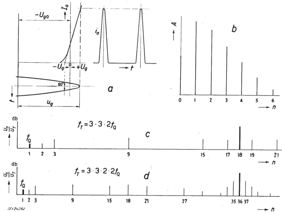
Fig. 3 Frequenzvervielfachung grundsätzlich und in der Anwendung
