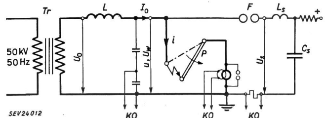
Fig. 12 Wechselstrom-Lichtbogen mit Stoss überlagert Schema der Anordnung Tr Transformator; P Pendel; F Funkenstrecke; L Drosselspule ( 5,2 \mu\text{H} ); C_s Stosskondensator ( 1 \mu\text{F} ); L_s Induktivität des ganzen Stosskreises ( 145 \mu\text{H} ); KO Kathodenstrahloszillograph; u gemessene Spannung (am Lichtbogen); U_0 Leerlaufspannung (31 kV); U_w wiederkehrende Spannung bei offenem Pendel und gezündeter Funkenstrecke F (46 kV); U_s Ladespannung des Stosskondensators (150 kV); i Lichtbogenstrom; I_0 Wechselstrom bei geschlossenem Pendel (19 A)
