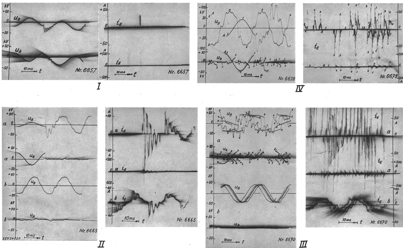
Fig. 20 Erdschluss durch rissige Isolatoren Oszillogramm-Beispiele
