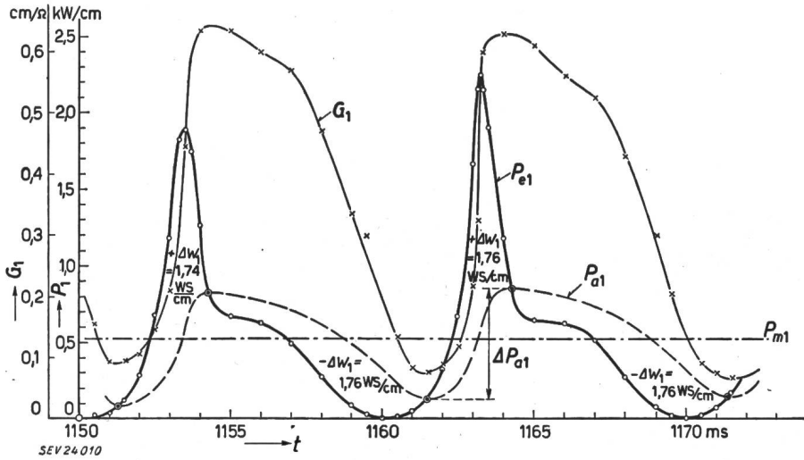
Fig. 10 Zeitlicher Verlauf der Leistungen und der Leitfähigkeit des Lichtbogens in ruhender Luft VG 3: U_0 = 31 kV, U_w = 46 kV I_0 = 19 A, C = 1 \mu\text{F} Lichtbogenlänge 346 cm, Osz. Nr. 3204 (Fig. 7b, Kurve III) P_{e1} eingeführte Leistung pro cm Lichtbogenlänge P_{a1} abgeführte Leistung pro cm Lichtbogenlänge P_{m1} mittlere Leistung G_1 Leitfähigkeit des Lichtbogens pro 1 cm \Delta W_1 Änderung der in 1 cm Lichtbogen aufgespeicherten Energie, welche die abgeführte Leistung um \Delta P_{a1} ändern lässt (Fläche zwischen P_{e1} und P_{a1} )
