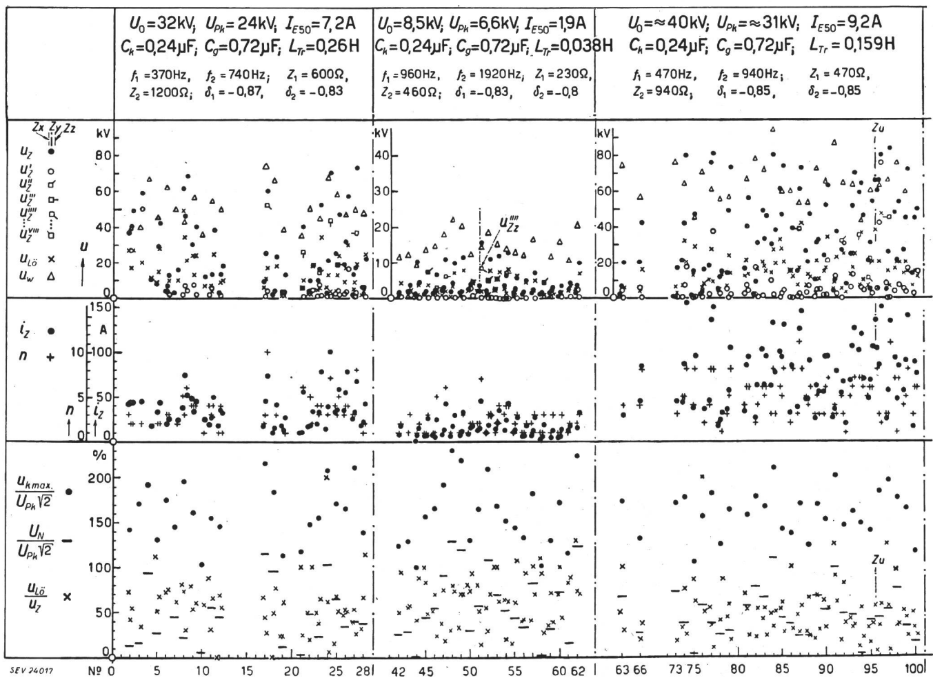
Fig. 17 Erdschluss mit Lichtbogen in Öl Zusammenstellung der Resultate
