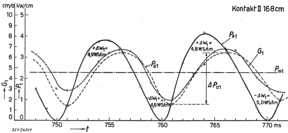
Fig. 11 Zeitlicher Verlauf der Leistungen und der Leitfähigkeit des Lichtbogens in ruhender Luft VG 6: U_0 \approx U_w = 31 kV, I_0 = 116 A, C = 0,004 \mu\text{F} Lichtbogenlänge 168 cm Osz. Nr. 3294 (Fig. 9b, Kurve II) Weitere Bezeichnungen siehe Fig. 10
