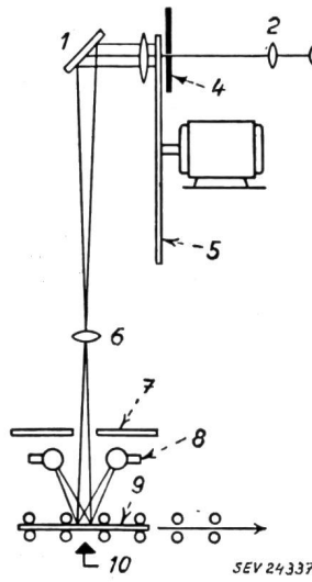
Fig. 1 Optisches System zum Lesen einer Textzeile 1 Spiegel; 2 Linse; 3 Vervielfacher-Photozelle; 4 Platte mit waagrechttem Schlitz; 5 rotierende Abtastscheibe; 6 Objektiv; 7 Abdeckmaske; 8 Beleuchtung; 9 Schriftstück; 10 Lesestelle
