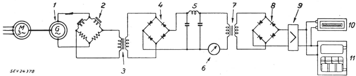
Fig. 2 Prinzipischema der Exzentrizitätsmessung
