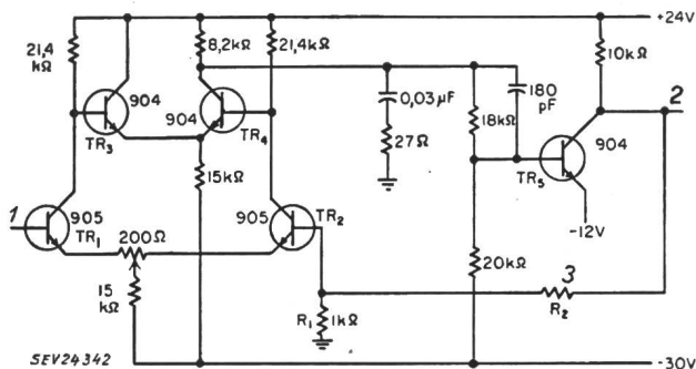
Fig. 2 Stabiler Gleichstromverstärker mit npn-Transistoren 60 db Spannungsverstärkung 1 Eingang; 2 Ausgang; 3 Gegenkopplung
