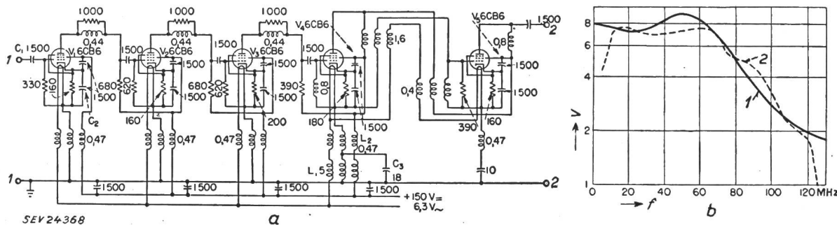
Fig. 3 Fünfstufiger Allpass-Verstärker
