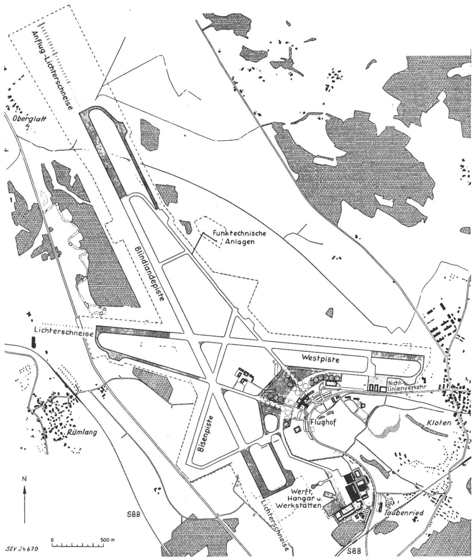
Fig. 1 Interkontinentaler Flughafen Zürich-Kloten Lageplan; 1. und 2. Bauetappe 1. Bauetappe: bestehende Anlagen □ Pisten und Rollwege, Flugsteig ■ Gebäude 2. Bauetappe: projizierte Anlagen □ Pisten und Rollwege, Flugsteig □ Gebäude
