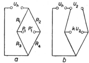
Fig. 9 Zerlegung der Schaltung in Fig. 8
