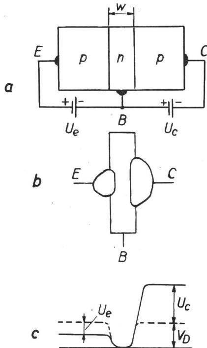
SEV 24839 Fig. 12 p-n-Transistor
