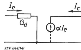
Fig. 13 Vereinfachtes Ersatzschema des Transistors I_e Emitterstrom; I_c Kollektorstrom; G_d Leitwert des Emitter-Überganges; \alpha Stromverstärkungsfaktor
