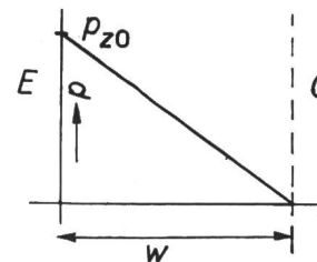
Fig. 14 Konzentrationsverlauf in der Basis des Transistors E Emitter; B Basis; C Kollektor; p Löcherkonzentration; p_{z0} Überschusslöcherkonzentration beim Emitterübergang; w Basisbreite
