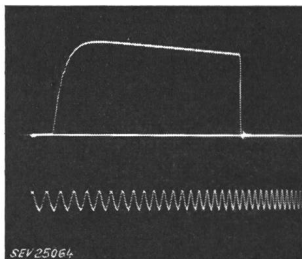
Fig. 5 Nach 9 \mu\text{s} abgeschnittene Stossweite Eichfrequenz 2 MHz
