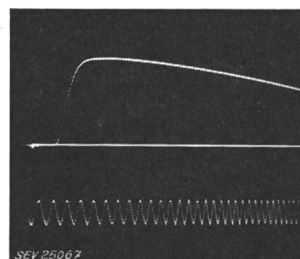
Fig. 8 Vollwelle des 1-MV-Stossgenerators Scheitelwert 1020 \text{ kV} Eichfrequenz 2 MHz
