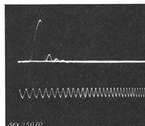
Fig. 11 Stosswelle des Holzspaltens Eichfrequenz 2 MHz
