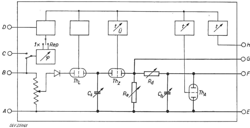
Fig. 2 Blockschema des Repetitions-Stossgenerators Eingänge: A Netz; B Netz; C Steuerfrequenz; D Fremdimpuls Ausgänge: E Erde; F Stosswelle; G Zündimpuls; H Oszillographimpuls Stosskreiselemente: C_s Stosskapazität; R_e Entladewiderstand; R_d Dämpfungswiderstand; C_b Belastungskapazität; Th_L Ladethyatron; Th_Z Zündthyatron; Th_A Abschneidethyatron; U Überbrückungsschalter; t Zeiteinstellungen; \varphi Phasenregelung; 1 \times einmalige Auslösung; Rep wiederholte Auslösung
