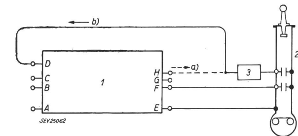
Fig. 3 Schaltung: Repetitions-Stossgenerator mit Kathodenstrahl-Oszillograph 1 Repetitions-Stossgenerator; 2 Kathodenstrahl-Oszillograph; 3 Zeitablenkung; D Eingang Fremdimpuls; E Ausgang Erde; F Ausgang Stosswelle; H Ausgang Oszillographimpuls a) Variante a; b) Variante b Weitere Bezeichnungen siehe in Fig. 2
