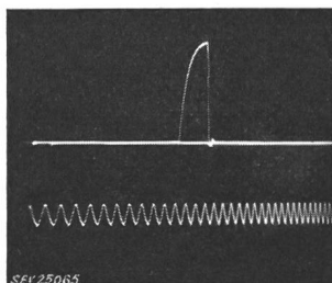
Fig. 6 Nach 1 \mu\text{s} abgeschnittene Stossweite Eichfrequenz 2 MHz
