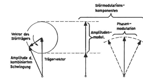
Fig. 3 Störcharakteristik eines diskreten unmodulierten Störträgers 100% Phasenmodulation sei \pm 1 rad, d. h. eine Phasenabweichung, die dasselbe Frequenzband beansprucht wie eine amplitudenmodulierte Übertragung mit identischem Nachrichteninhalt
