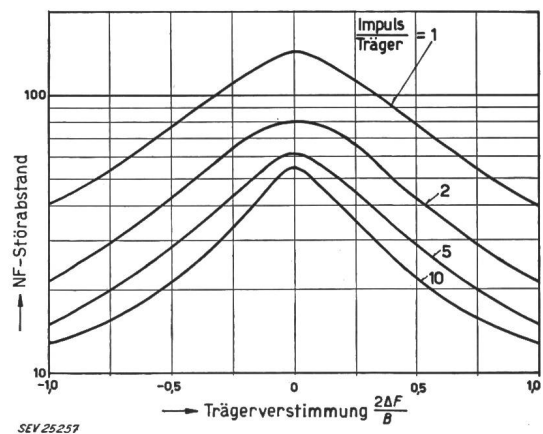
Fig. 5 NF-Störabstand bei Impulsstörungen eines FM-Empfängers als Funktion der Trägerverstimmung gegen die Bandmitte 1300 Störimpulse/s
