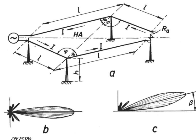
Fig. 1 Schema der Rhombusantenne HA Hauptachse; h Höhe der Antenne Weitere Erklärungen siehe im Text
