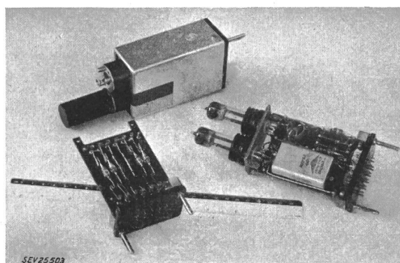
Fig. 3 Steckbare Einheiten
