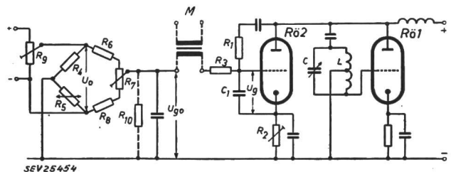
Fig. 1 Grundschemata der Temperaturkompensation mittels Reaktanzröhre C, L Schwingkreis; Rö1 Schwingröhre; Rö2 Reaktanzröhre Weitere Bezeichnungen siehe im Text
