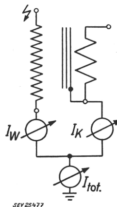
Schema der Stromerfassung bei der Stossprüfung von Transformatoren
