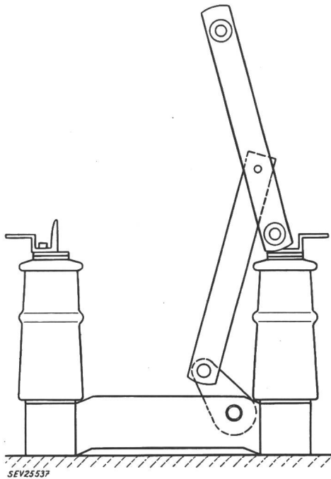
Fig. 4 Innenraum-Trennschalter
