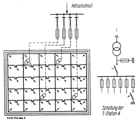
Fig. 2 Mehrstranggespeistes Niederspannungs-Maschennetz mit in der Werkhalle aufgestellten S(Speise)-Stationen
