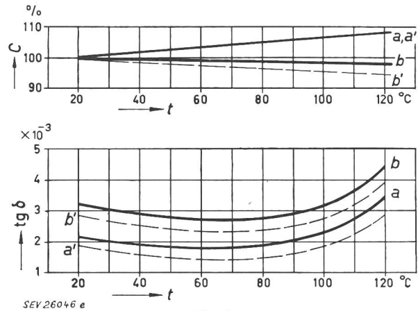
Fig. 4 Verlustfaktor \text{tg } \delta und Kapazität C von Papieren verschiedener Satinage in Funktion der Temperatur a vakuumgetrocknete, unimprägnierte Wickel, Satinage A b mit Pyralene 1476 imprägnierte Wickel, Satinage A a' vakuumgetrocknete, unimprägnierte Wickel, Satinage C b' mit Pyralene 1476 imprägnierte Wickel, Satinage C
