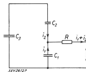
Fig. 4 Kapazitive Anordnung zur Berechnung des Energieabfalles R Oberflächenwiderstand des Spaltes und Widerstand der Entladungsbahn; i_1 , i_2 Übergangsströme bei der Entladung Weitere Bezeichnungen siehe Fig. 2
