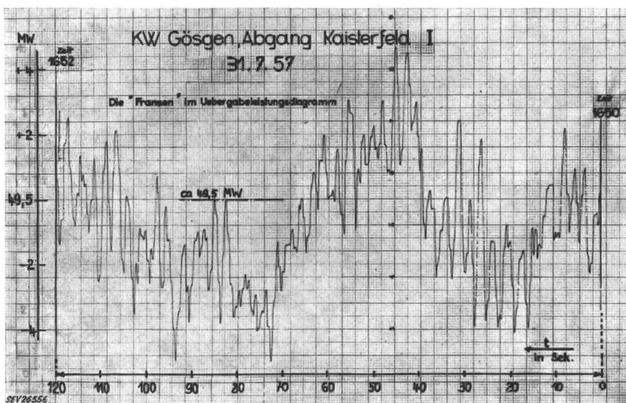
Fig. 14 Diagramm der Übergabeleistung im Kraftwerk Gösgen, Feeder Kaiserfeld, aufgenommen mit Funktionschreiber (Nullpunkt unterdrückt)
