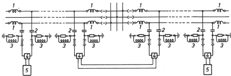
Fig. 10 Ausrüstung von 2 HF-Teilstrecken mit Zweiphasenkopplung, welche über eine Hochfrequenzbrücke verbunden sind 1 Sperre; 2 Kopplungskondensator; 3 Ableiter und Erdungsdrosselspule; 4 Koppelfilter; 5 Trägerfrequenzausrüstung
