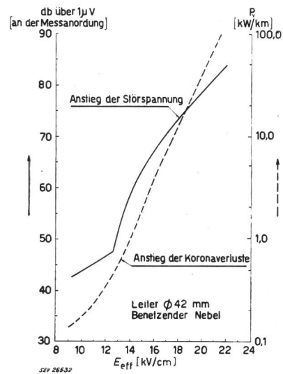
Fig. 2 Anstieg der HF-Störspannung und der Koronaverluste P_v für einen bestimmten Leiter in Funktion der Feldstärke E an der Leiteroberfläche
