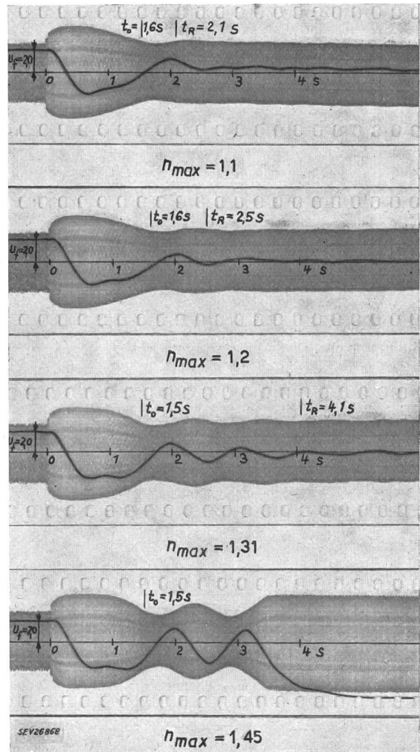
Fig. 18 Spannungsregelung mit Verstärkermaschine Lastabwurf mit Drehzahlanstieg, c = 0,6 n_{max} auf Nennzahl bezogene max. Drehzahl Weitere Bezeichnungen s. Fig. 15
