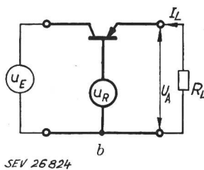
Fig. 1 Einfache Stabilisierungsschaltungen a mit Quertransistor; b mit Längstransistor
