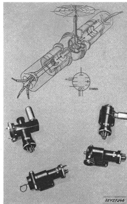
Fig. 12 Klystron
