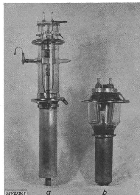
Fig. 7 Senderöhren
