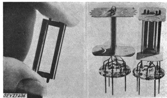
Fig. 2 Rahmen-Gitter
