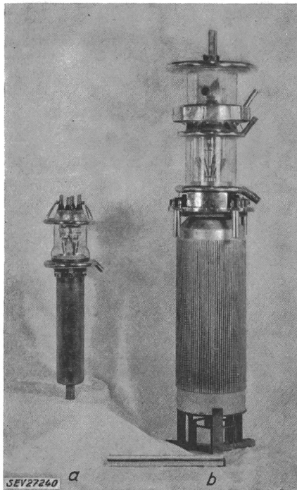
Fig. 6 Senderöhren
