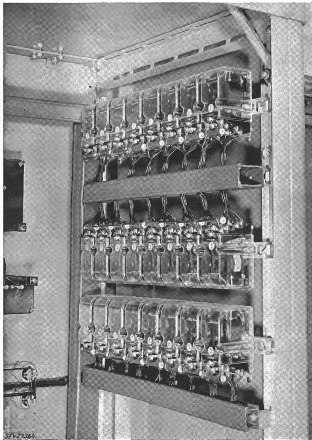
Fig. 4 Kanalverdrahtung
