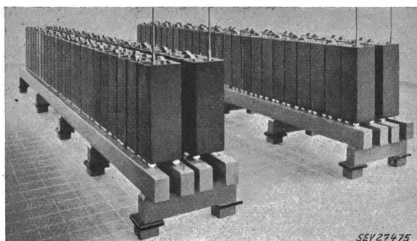
Fig. 3 Stationäre Batterie Typ PAM, bestehend aus Einzelementen
