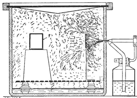
Fig. 9 Caisse fermée et vaporisateur pour l'essai de résistance à l'humidité
