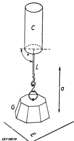
Fig. 7 Sollicitation de conducteurs de raccordement à la traction C Condensateur L Conducteur de raccordement G Poids de charge E Support plan, en feutre a Course de levage (= 10 cm)
