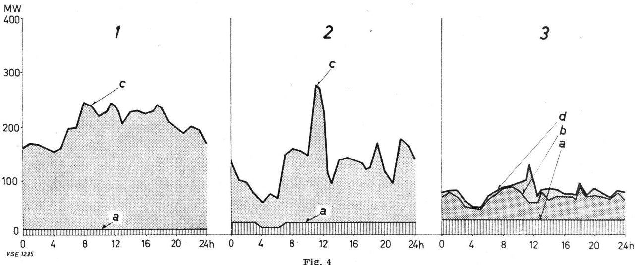
Charges horaires du réseau de l'EOS à différentes périodes de l'année 1958
