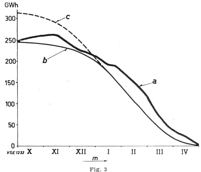
Statistique de l'utilisation de l'énergie accumulée. Année 1954/55 Compensation de l'insuffisance du remplissage des bassins d'accumulation par très forte réduction des prélèvements d'énergie accumulée, en octobre et novembre
