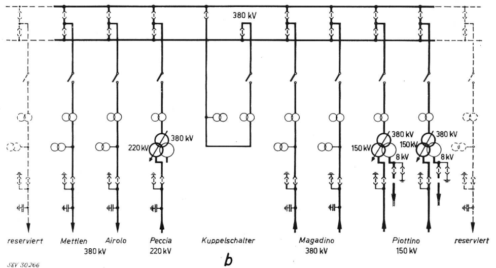
Fig. 2 Einpoleiges Schema der Station Lavorgo a Ausbau 220 kV; b Ausbau 380 kV
