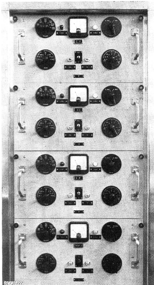
Fig. 2 Etage de manipulation duplex Centre émetteur de Prangins
