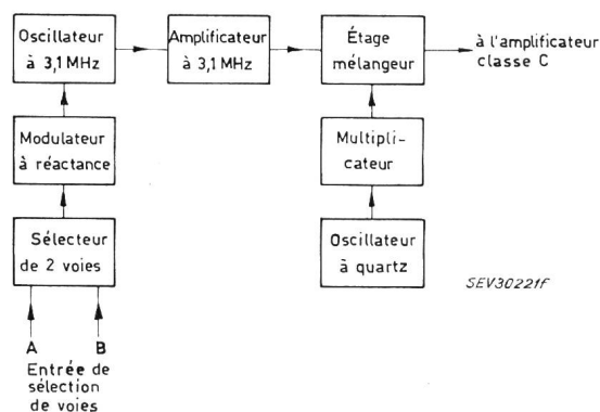
Fig. 1 Etage de manipulation duoplex
