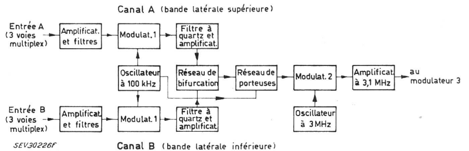
Fig. 6 Générateur de bande latérale unique pour la préparation de six voies multiplex à division dans le temps
