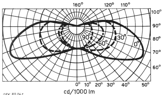
Fig. 3 Lichtverteilung einer Leuchte mit nichtrotationssymmetrischem Lichtbündel Polardiagramme der Ebenen 0°, 30°, 60° und 90°
