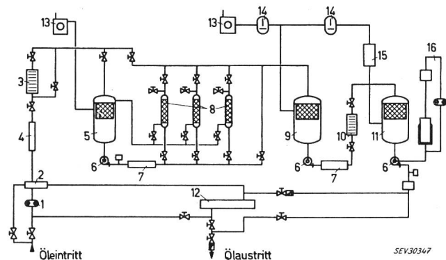
Fig. 10 Kombinierte Aufbereitungs- und Regenerierungs-Anlage 1 Förderpumpe; 2 Mengenregler; 3 Filterpresse; 4 Kühler; 5 Entgasungskessel 1. Stufe; 6 Umwälzpumpen; 7 Ölwärmer 25 kW; 8 Fuller-Kessel; 9 Entgasungskessel 2. Stufe; 10 Filterpresse; 11 Entgasungskessel 3. Stufe; 12 Ölwärmer 120 kW; 13 Drehschieberpumpen S = 100 \text{ m}^3/\text{h} ; 14 Rootspumpen S = 1600 \text{ m}^3/\text{h} ; 15 Kondensator; 16 Inhibieranlage
