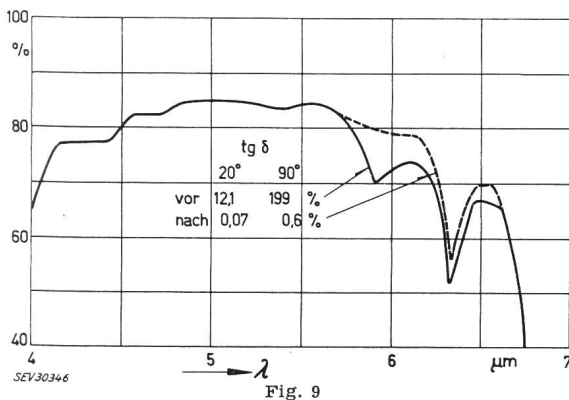
Fig. 9 IR-Spektren (Ausschnitte) eines stark gealterten Öls vor und nach der Regeneration \lambda Wellenlänge
