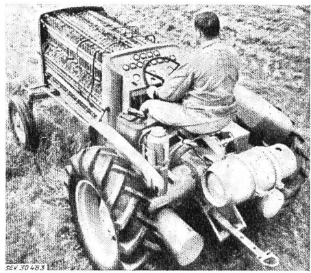
Fig. 5 Ansicht des elektrochemisch angetriebenen Traktors der Allis-Chalmers Mfg. Co. Unter dem Führersitz befindet sich das Stahlfass mit dem Brenngas H_2 + C_2H_6 , unter dem Fahrzeug Druckflaschen mit O_2 -Kraftregelung und Rückwärtsgang durch Controller Höchstleistung 15 kW
