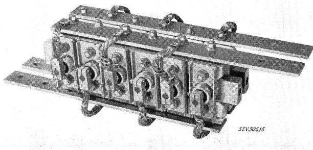
Fig. 15 Silizium-Gleichrichtergruppe für Wasserkühlung
