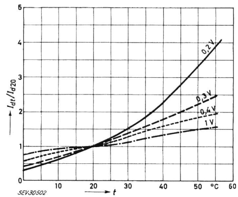
Fig. 2 Temperaturverhalten des Durchlaßstromes einer Kupferoxydulzelle
