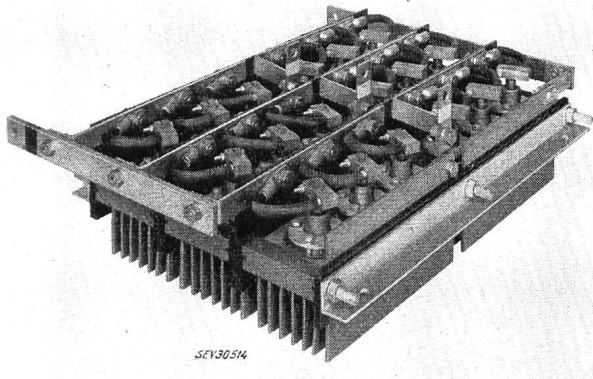
Fig. 14 Silizium-Gleichrichtergruppe für Ventilator Kühlung
