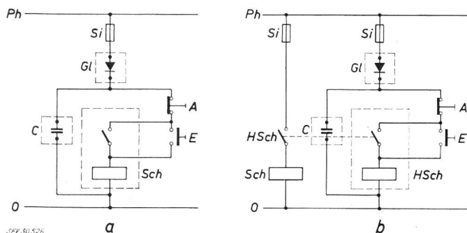
Fig. 1 Steuerstromkreise
