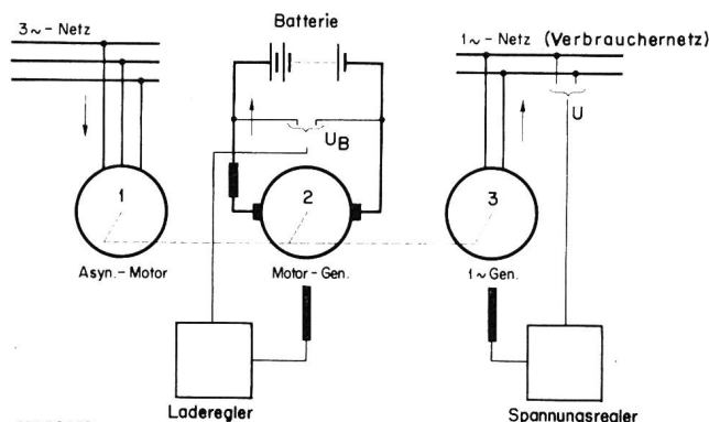
Fig. 1 Schema einer Energieversorgungsanlage im Normalbetrieb Speisung vom Netz 1 Antriebsmotor; 2 Motor-Generator; 3 Einphasengenerator; U_B Batteriespannung; U Verbrauchernetzspannung
