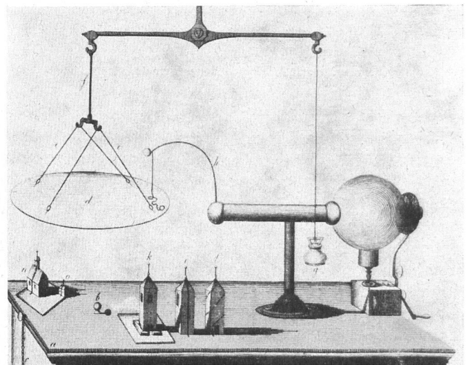
Fig. 6 Experiment 1781 zum Nachweis der Anziehungskraft einer Gewitterwolke sowie der Nützlichkeit eines Wetterableiters [6] a mit Zinnfolie beklebter Tisch; d mit Zinnfolie beklebte Tafel; e Seidenfäden; f Waagebalken; g Gegengewicht; i Turm mit Ableiter; k Turm ohne Ableiter; l Turm mit unterbrochenem Ableiter; n Kirche mit Ableiter; o Haus
