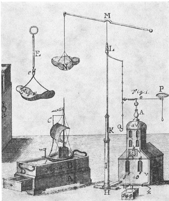
Fig. 5 Blitzmodellanlage aus 1780 [5]
