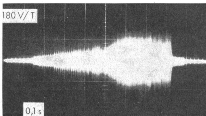
Fig. 1 Störsignal durch Trennerbetätigung gemessen am Hochfrequenzgang eines Einseitenband-Empfängers
