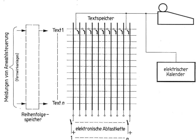
Fig. 8 Prinzipschema eines Informationsspeichers für die selbsttätige Protokolliereinrichtung
