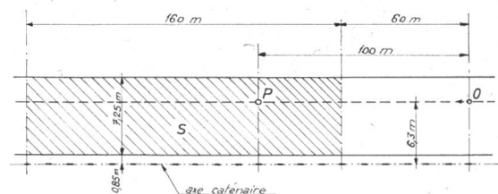
Fig. 8 Renseignements demandés au constructeur relatifs aux luminances P Luminance ponctuelle; S Luminance moyenne; O Observateur Hauteur d'observation = 1,50 m au-dessus du sol
