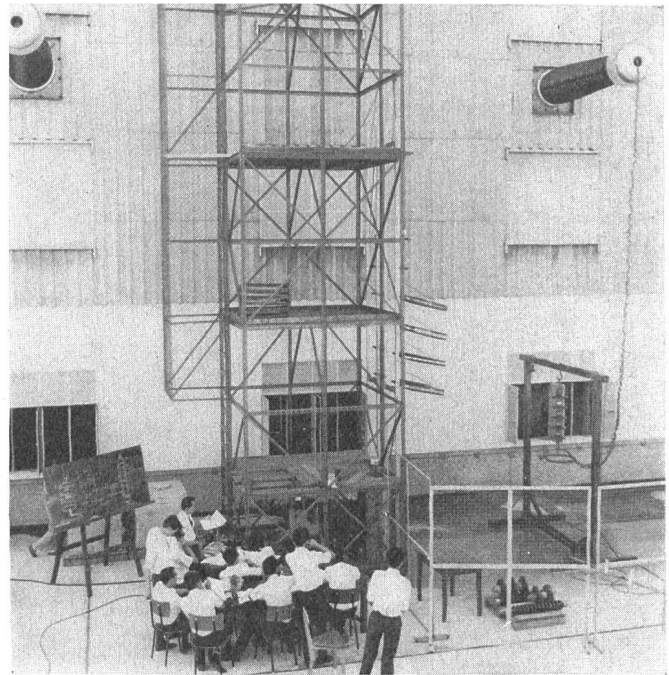
Fig. 13 Freiluftanlage, Versuche mit künstlichem Regen
