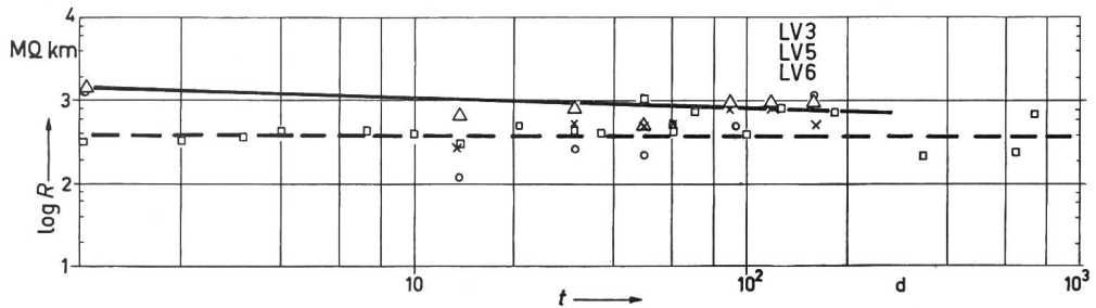
Fig. 21 Wie Fig. 20, aber fur Polyurethanlackdrahnte —△— Versuch LV 3 bei 20 °C und 95 % relative Luftfeuchtigkeit (RF); —□— Versuch LV 3 bei 70 °C und 95 % RF; —○— Versuch LV 5 bei 20 °C und 95 % RF; —×— Versuch LV 6 bei 20 °C und 95 % RF t Zeit
