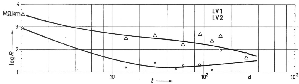
Fig. 20 Isolationswiderstand von Acetallackdrahnten in Abhangigkeit von einer Langzeitlagerung in feuchter Atmosphare —○— Versuch LV 1 bei 20 °C und 95 % relative Luftfeuchtigkeit (RF); —△— Versuch LV 2 bei 20 °C und 95 % RF
