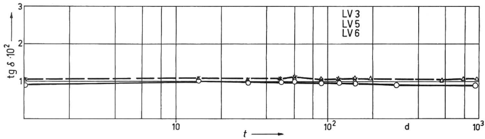
Fig. 19 Wie Fig. 18, aber fur die Polyurethangruppe —△— Versuch LV 3 bei 70 °C und 95 % relative Feuchtigkeit (RF); —○— Versuch LV 5 bei 20 °C und 95 % RF; —×— Versuch LV 6 bei 20 °C und 95 % RF t Zeit
