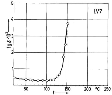
Fig. 6 Lackdrähte der Polyester-Gruppe Versuch LV 7
