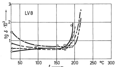
Fig. 15f Versuch LV 8
