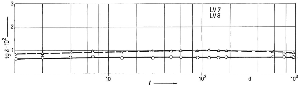
Fig. 22 Verlustwinkel von Lackdrähten der Polyester- bzw. Polyesterimidgruppe bei 1 kHz in Abhängigkeit von einer Langzeitlagerung in feuchter Atmosphäre —△— Versuch LV 7 bei 70 °C und 95 % relative Feuchtigkeit (RF); —○— Versuch LV 8 bei 70 °C und 95 % RF t Zeit
