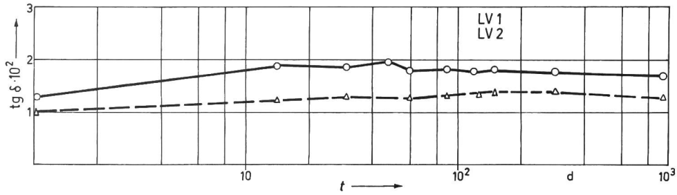
Fig. 18 Verlustwinkel \text{tg } \delta von Lackdrahnten der Polyvinylacetalgruppe bei 1 kHz in Abhangigkeit von einer Langzeitlagerung in feuchter Atmosphare —○— Versuch LV 1 bei 20 °C und 95 % relative Feuchtigkeit (RF); —△— Versuch LV 2 bei 20 °C und 95 % RF t Zeit
