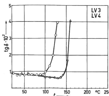
Fig. 4 Lackdrähte der Polyurethan- bzw. der Polyurethan-Polyamid-Gruppe —○— Versuch LV 3 —△— Versuch LV 4
