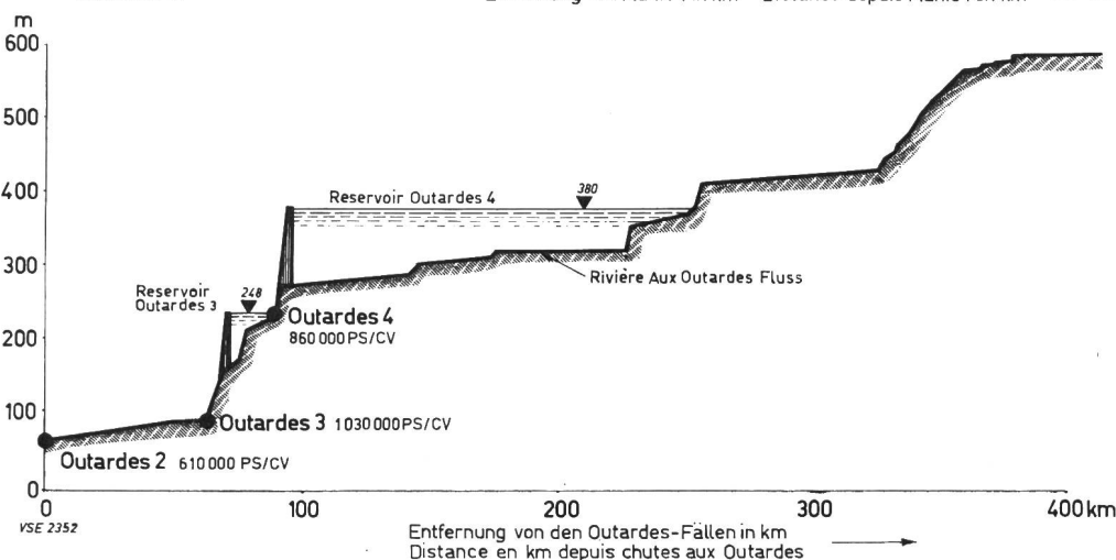
Fig. 11 Profil des rivières Manicouagan et Outardes
