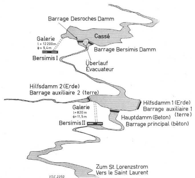
Fig. 7 Disposition des aménagements Bersimis I et II
