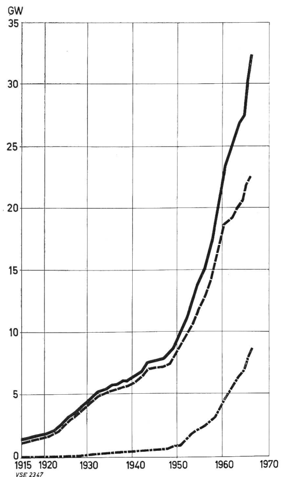
Fig. 1 Acroissement des puissances au Canada — Total - - - Hydro-électrique - · - · Thermique
