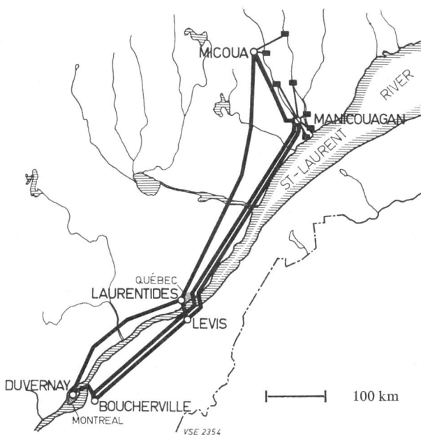
Fig. 17 Transport à 735 kV — Ligne ■ Centrale ○ Station
