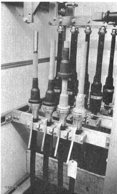
Fig. 5 Montage de garnitures terminales pour câbles PET
