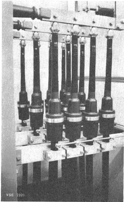
Fig. 4 Garnitures terminales de câbles d'alternateurs couplés en parallèle
