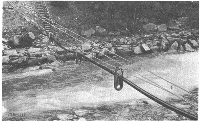
Fig. 6 Tirage d'un câble à travers la Reuss près d'Amsteg
