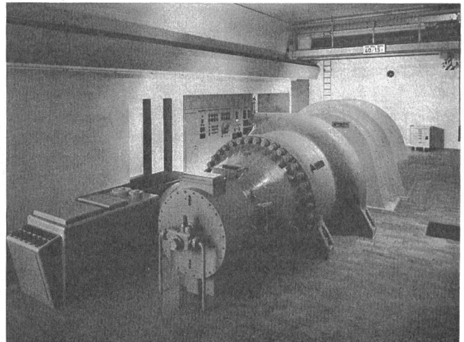
Fig. 5 Die dreistufige Pumpe mit dem Antriebsmotor
