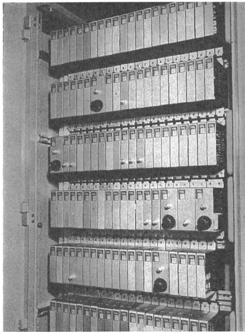
Fig. 19 Die kontaktlosen Steuerelemente der Anlaufautomatik
