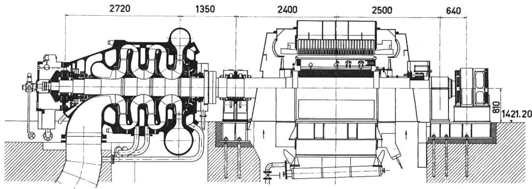
Fig. 7 Schnitt durch die Speicherpumpe und den Motor
