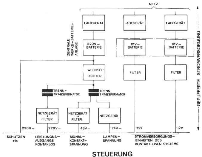
Fig. 27 Blockdiagramm der Energieversorgung für die Anlagen-Automatik
