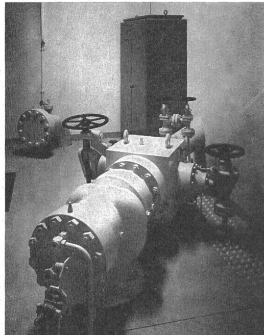
Fig. 8 Druckregler mit Steuerschrank an der Furnoleitung
