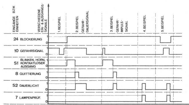
Fig. 22 Funktionsdiagramm eines elektrischen Gefahrenmelders
