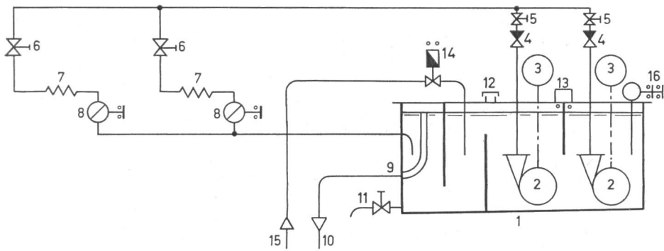
Fig. 11 Schema des Stehlagler-Kühlsystems
