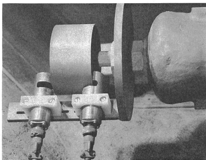
Fig. 21 Anordnung von Initiatoren für die berührungslose Lageabstastung
