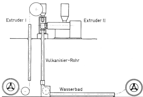
Fig. 12 CV-Vertikalanlage
