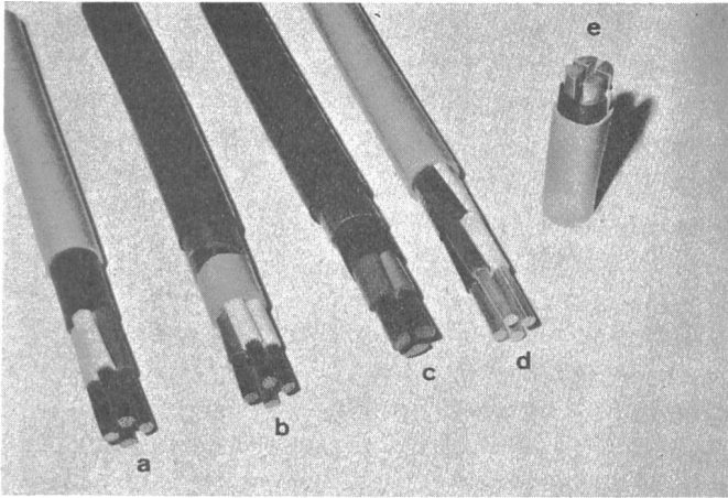
Fig. 5 TT (Tdc)-Kabel
