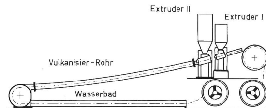
Fig. 13 CV-Schräganlage
