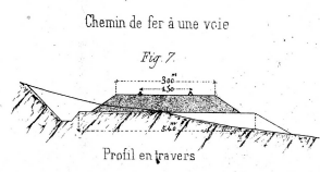
Profil en travers Fig. 7.
