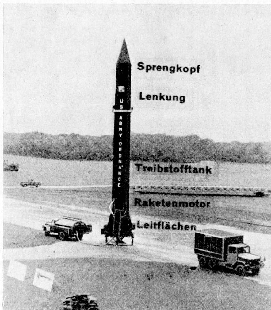
Abb. 4. Taktische Mittelstrecken-Lenkwaŕfe «Redstone» auf dem Abschußtiŕsch, kurz vor dem Senkrecht-Start
