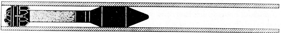
Rakete
