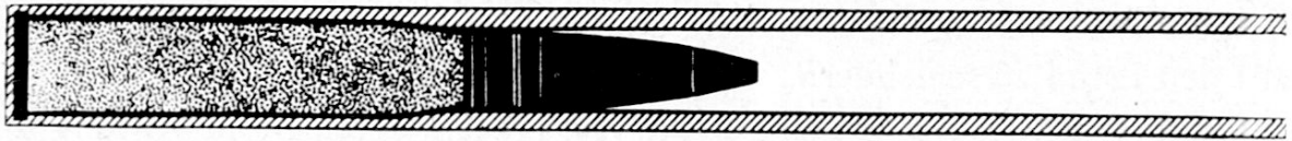
Klassische Kanone
