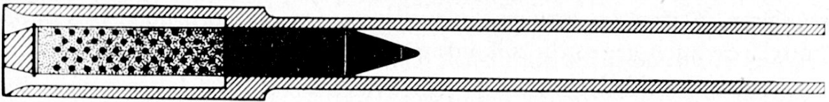
Rückstoßfreies Geschütz
