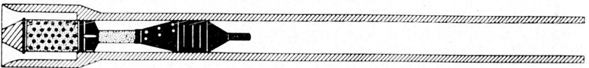
Geschütz-Rakete
