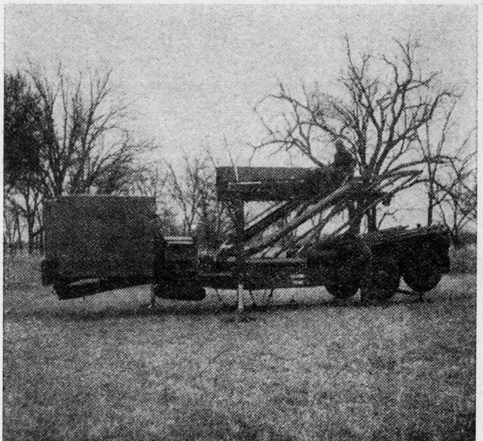
Bild 2 Abschußrampe im Aufbau, nach Abhängen des Schleppers
