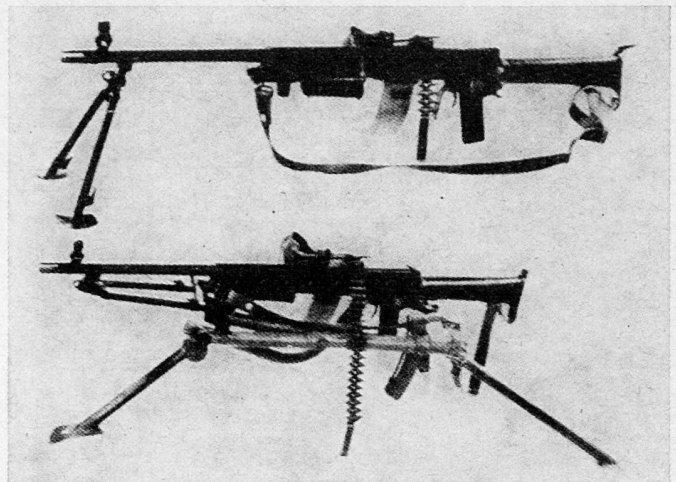
Maschinengewehr 60
